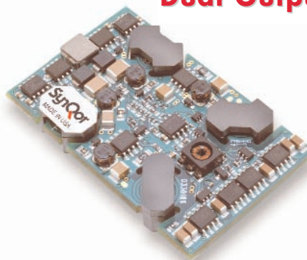
DQ63318QGL08 Module
